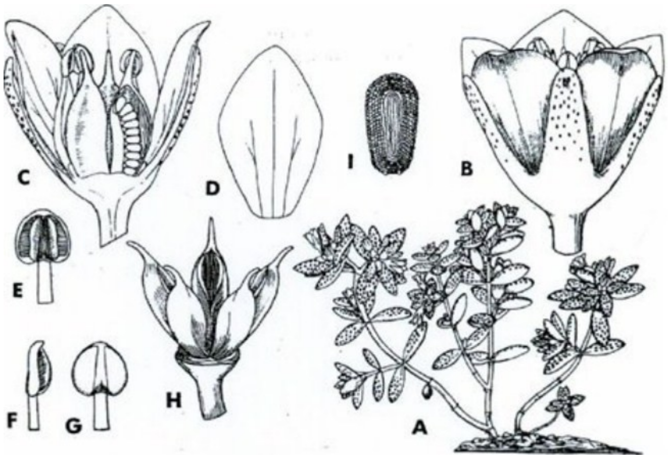
Fig. 1. - Crassula Humberti [Maintenant, Crassula humbertii ] : a, plante entière x 1 ; b, fleur entière x 10 ; c, coupe schématique de la fleur x 10 ; d, pétale isolé, à plat x 10 ; e, f, g, anthère vue de face, de profil, de derrière x 20 ; h, fruit, montrant les follicules (les restes desséchés du périanthe et de l'androcée ne sont pas figurés) x 10 ; i, graine X 30.
